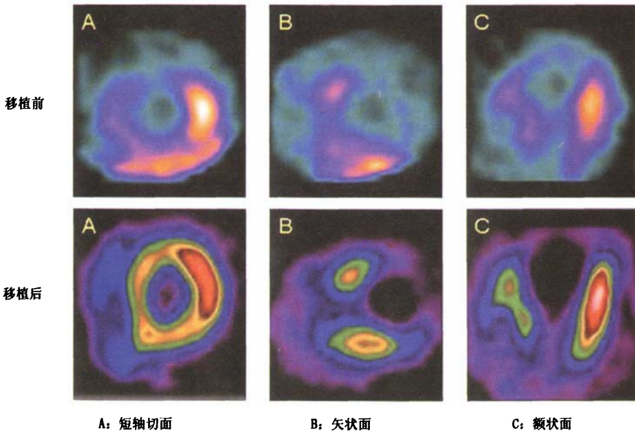
图 2 PBSC 移植前后 ^{99m}\text{Tc} -MIBI 心肌灌注显像
